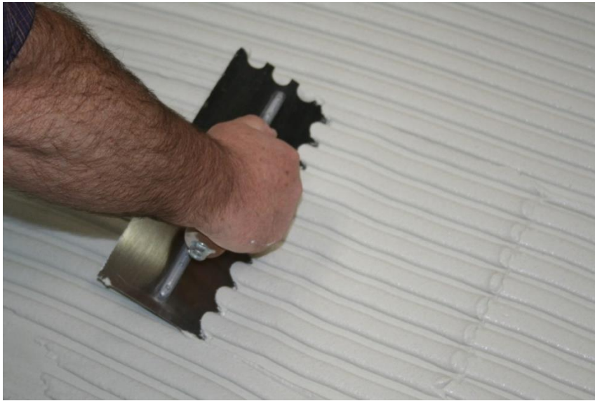
Picture 1.2 - \frac{3}{4} " (18mm) llana dentada con un mortero de capa media usada en baldosas de gran formato. Raye el mortero en una dirección tomando la llana en un ángulo de 45° grados. Note los canales de mortero que quedaron atrás.
